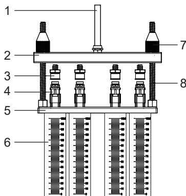
Diagramm zur Installation des oberen Kraftstoffinjektors
